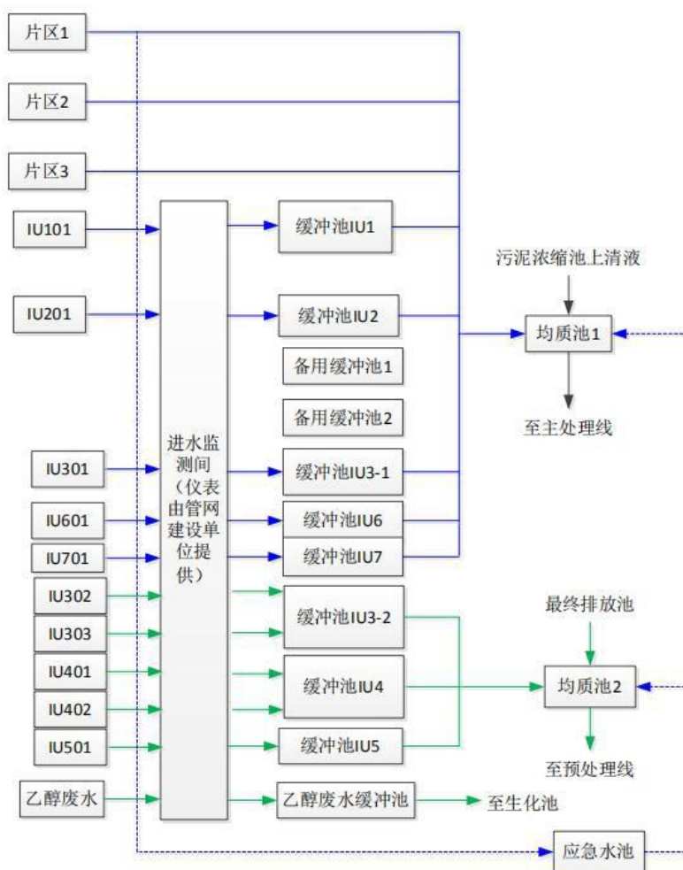
图 6.2-2 废水收集系统工艺流程图
