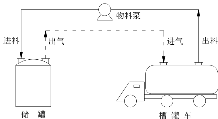
图 6.1.2-1 物料进入储罐时的无组织排放控制措施
