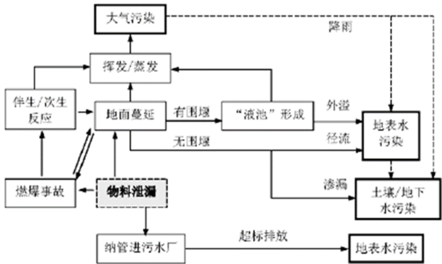
图 3.8-1 物料泄漏后环境扩散途径示意图
