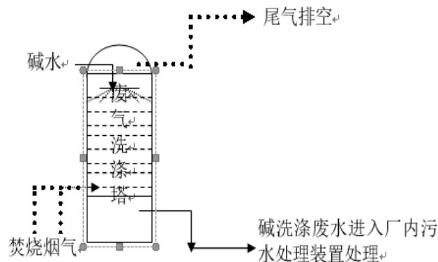
图 6.1.1-3 碱喷淋塔处理流程图
