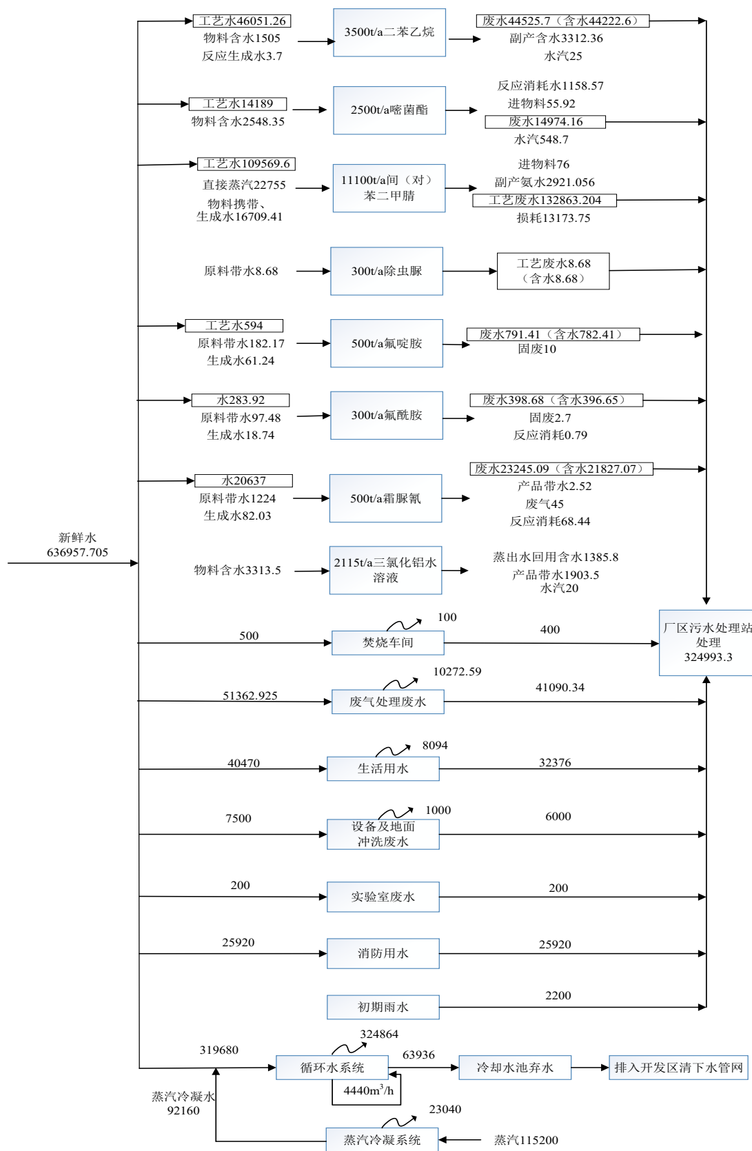
图 3.1.3-1 南厂区水平衡图 (单位: m³/a)
