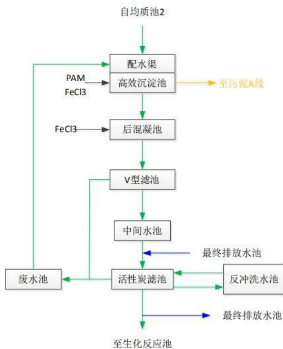
图 6.2-3 废水预处理系统工艺流程图
