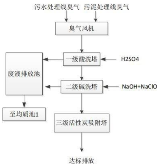
图 6.2-7 废水除臭系统工艺流程图
