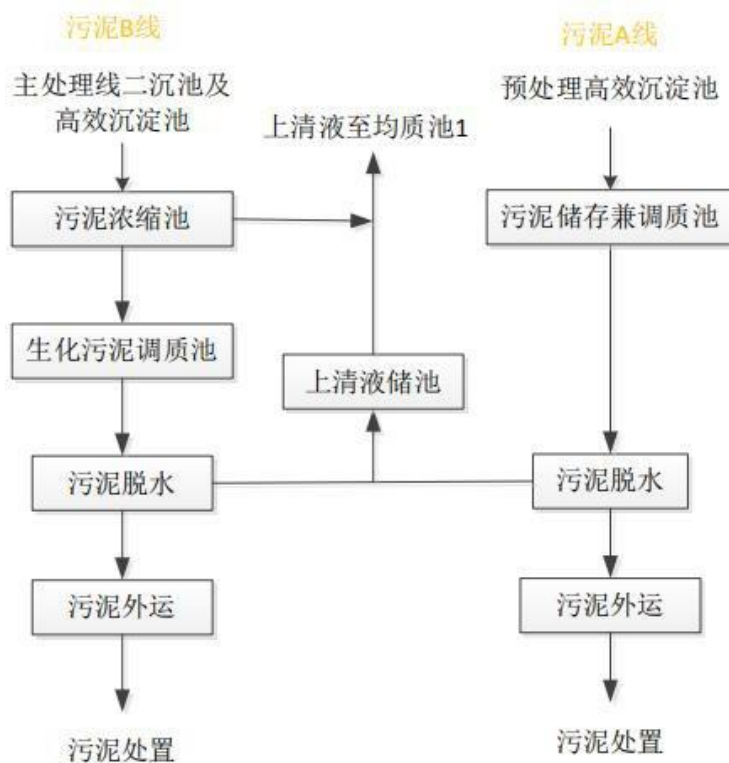
图 6.2-6 废水污泥处理系统工艺流程图
