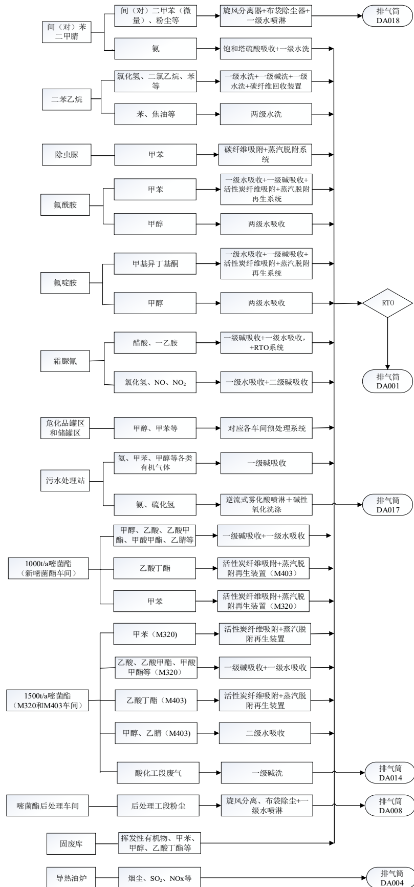
图 3.1.4-1 南厂区现有项目废气治理措施示意图
