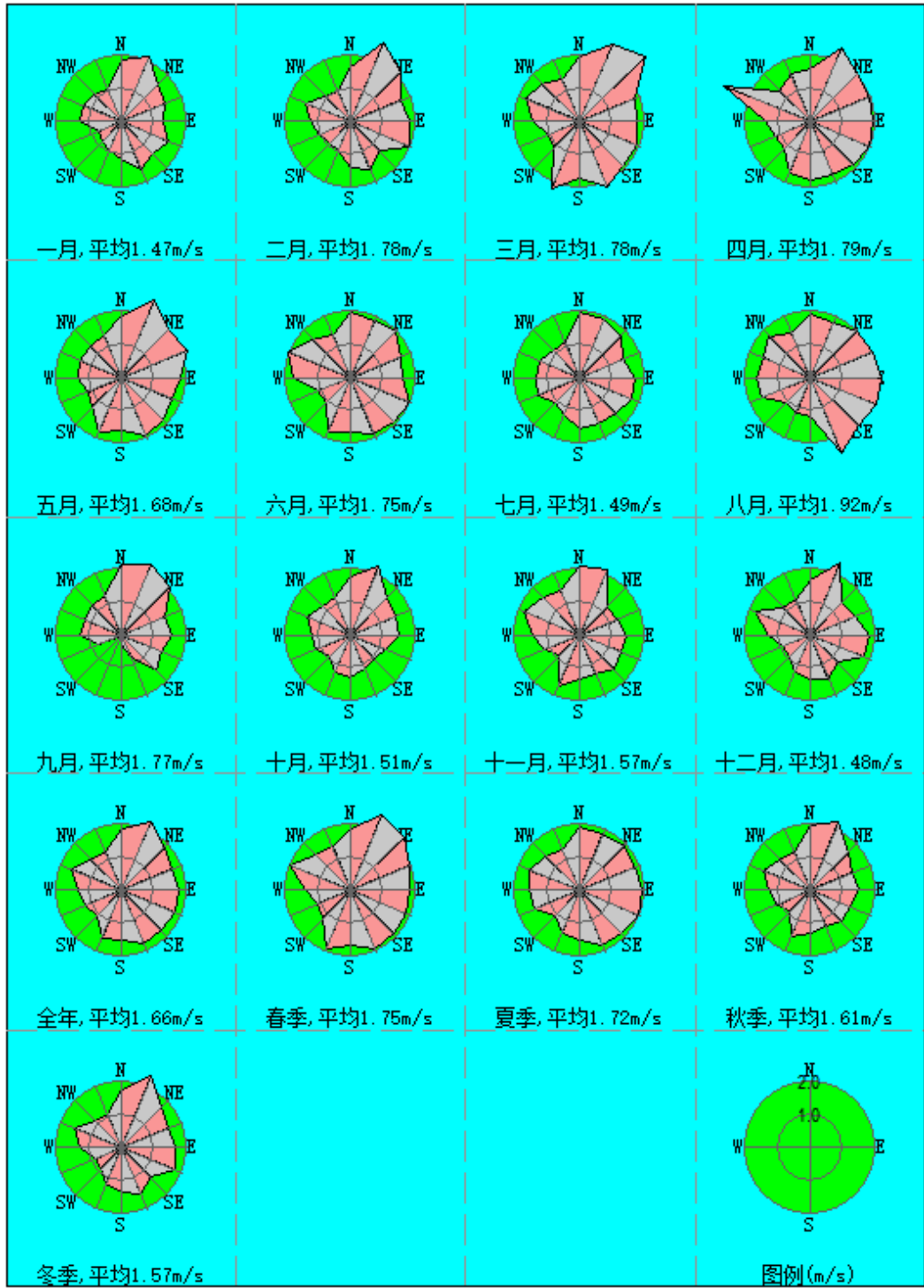
图 5.2.2-4 区域风玫瑰图
