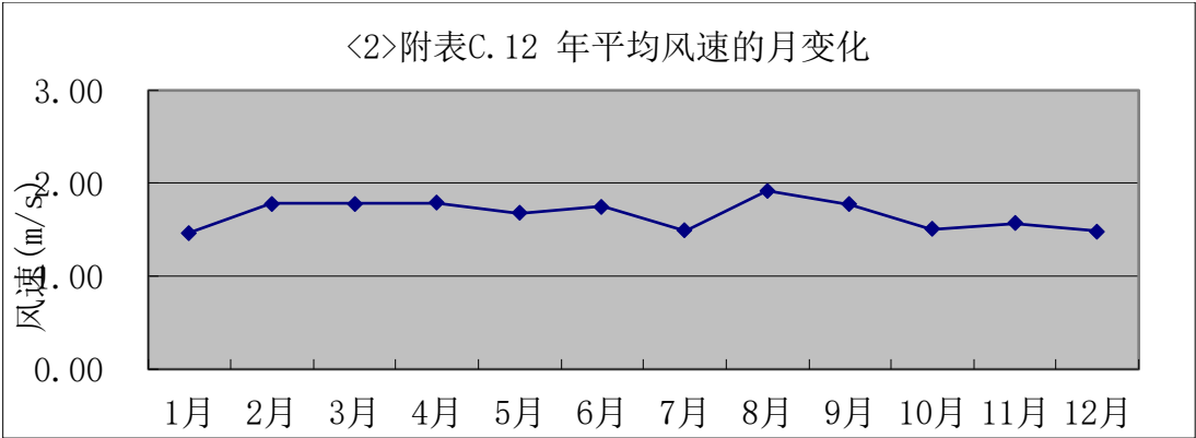
图 5.2.2-2 区域各月平均风速变化情况图
