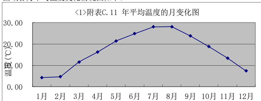
图 5.2.2-1 区域各月平均温度变化图
