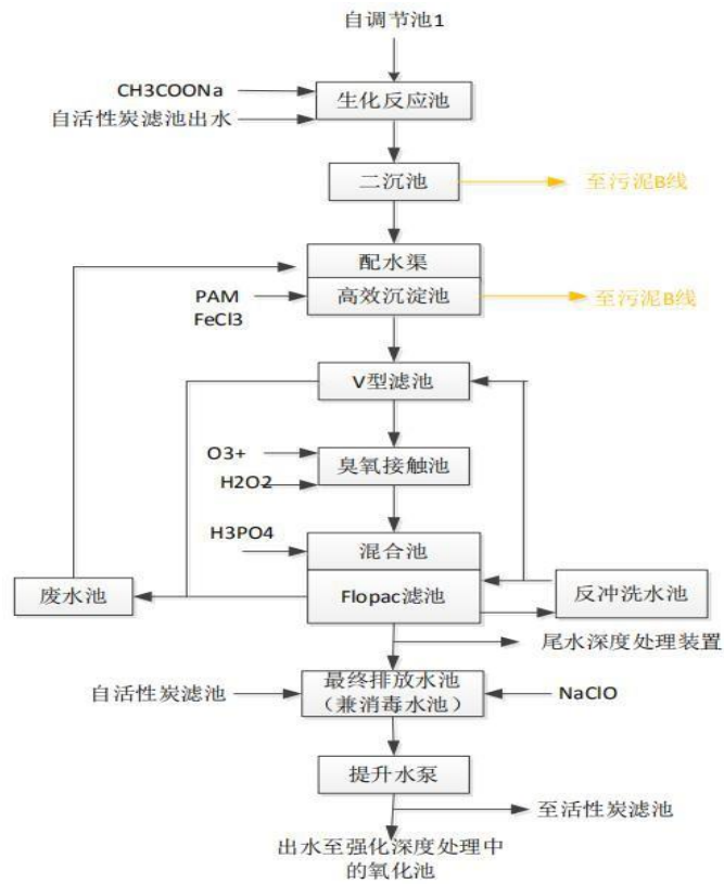
图 6.2-4 废水主处理工艺流程图
