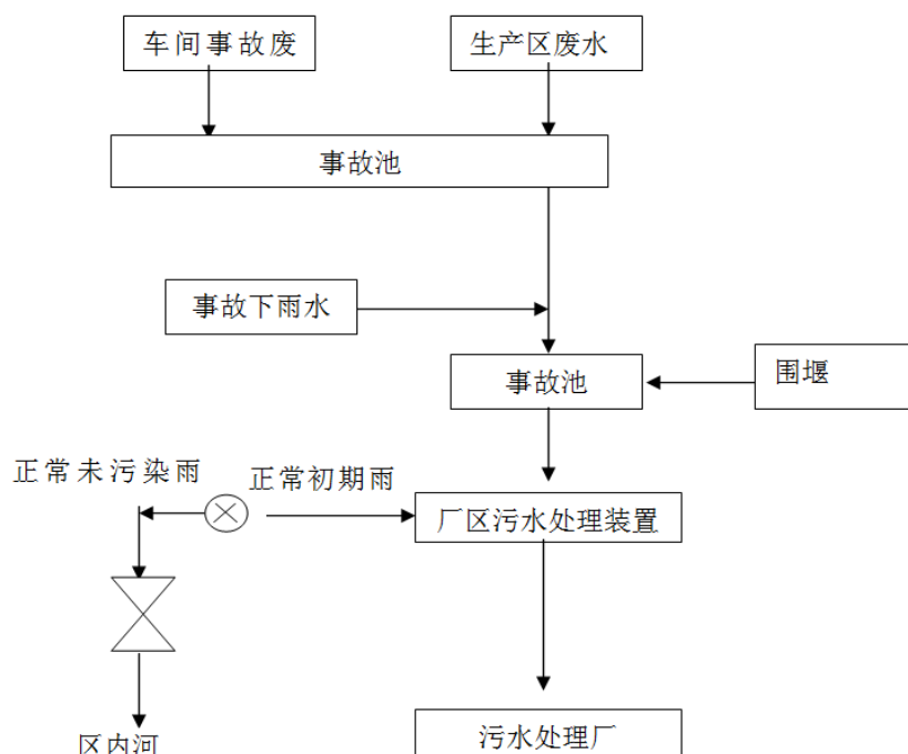
图 6.6-1 事故水收集系统示意图
