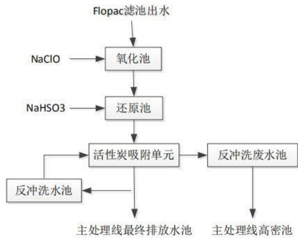
图 6.2-5 废水尾水深度处理提升装置工艺流程图
