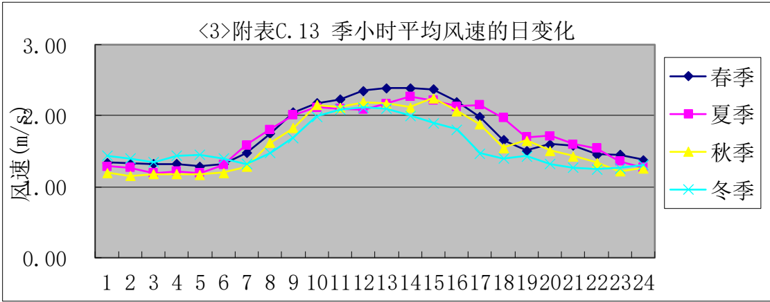
图 5.2.2-3 区域季小时平均风速的日变化情况图
