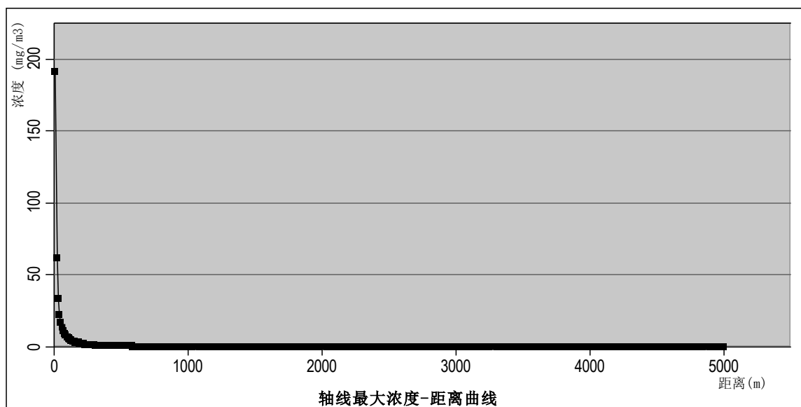
图 5.7.3-2 (2) 甲醇储罐泄漏常见气象条件下风向轴线最大浓度图
