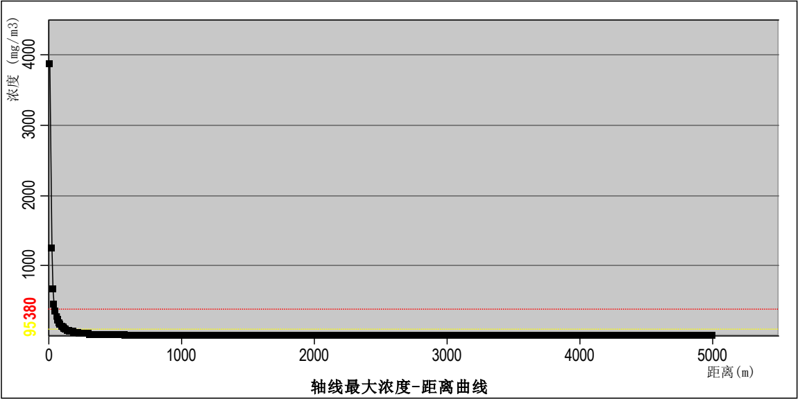
图 5.7.3-6（1） 次生 CO 最不利气象条件下风向轴线最大浓度图
