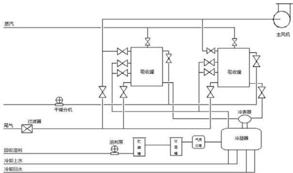
图 6.1.1-2 冷凝+碳纤维吸附处理工艺流程图
